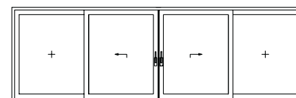
4-teiliges Element mit zwei Hebe-Schiebeflügeln und zwei Festverglasungen
