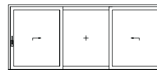
3-teiliges Element mit zwei Hebe-Schiebeflügeln und Festverglasung
