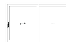
2-teiliges Element mit Hebe-Schiebeflügel und Festverglasung
