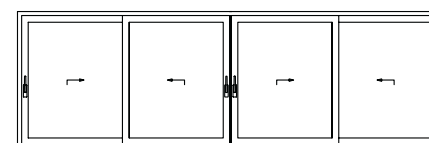
4-teiliges Element mit vier Hebe-Schiebeflügeln
